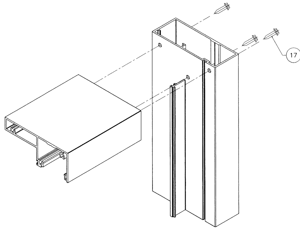
DOOR FRAME CORNER
